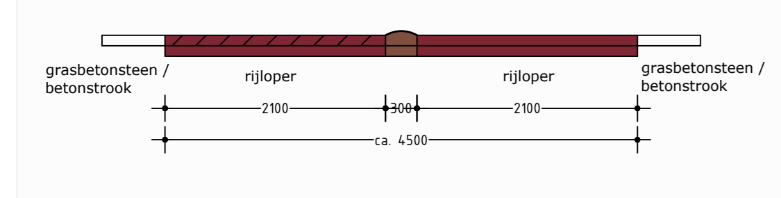
Principe doorsnede B-B fietsstraat Schaal 1:50
