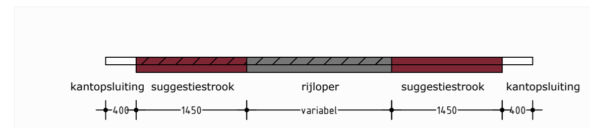
Principe doorsnede A-A fietsstroken Schaal 1:50
